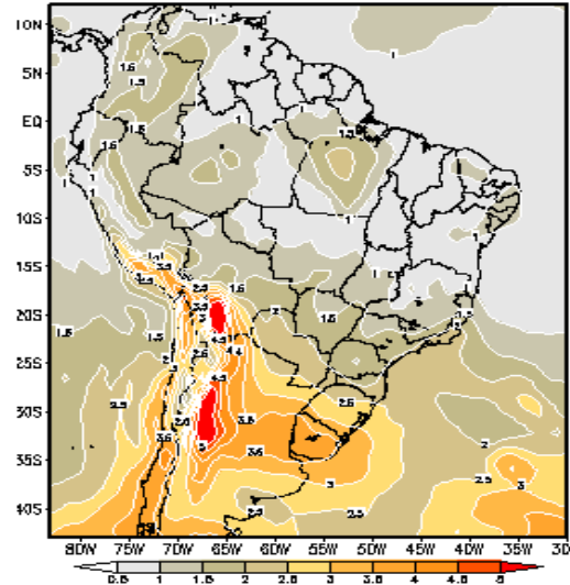
REQM de Pressão Reduzida ao NMM (mb) do T126 previsões para 48ha iniciadas as 00Z - Aug/2010
